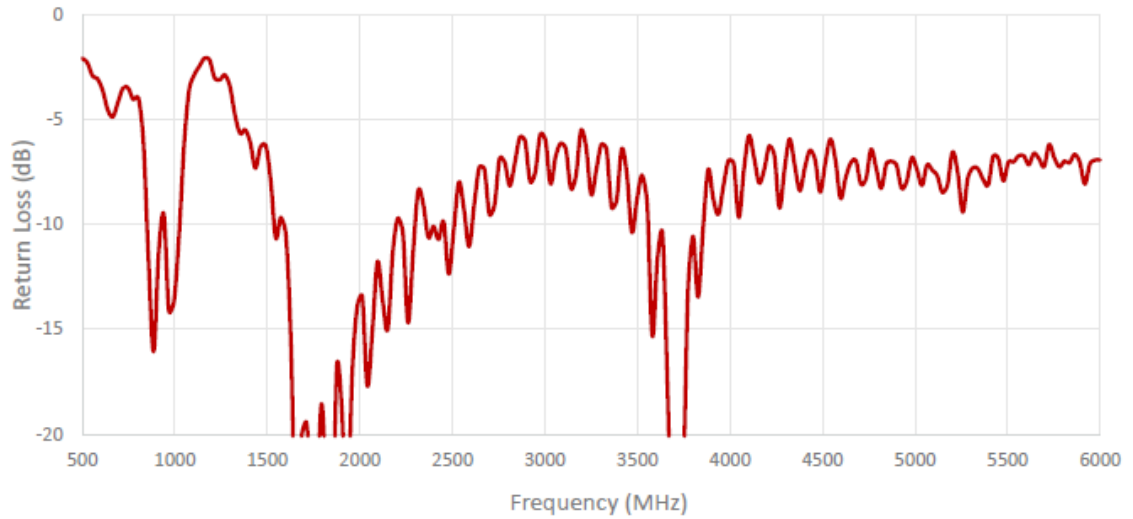
Cable 1: 5GNR
