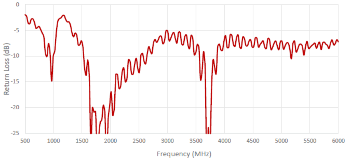
Cable 2: 5GNR
