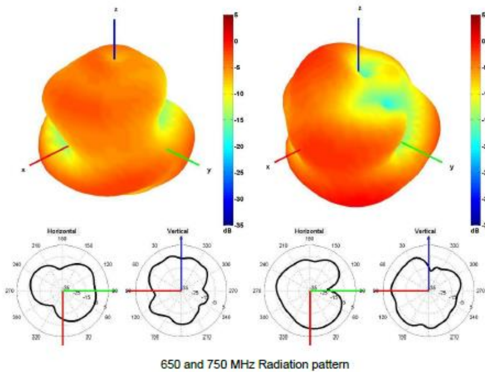
Cable 1: 5GNR
